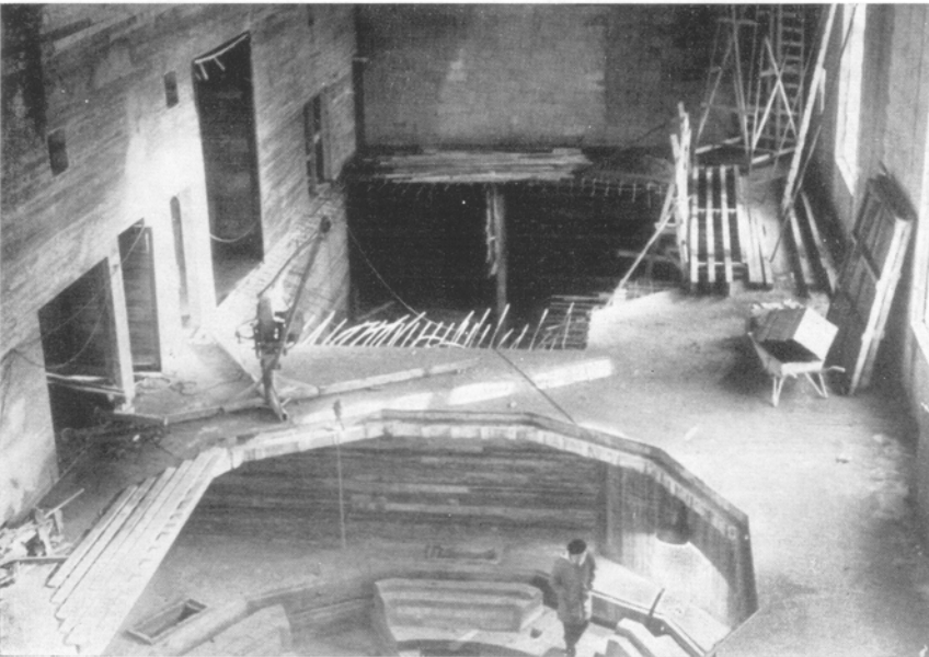
Stasjonsballen hvor generatoren skal plasseres. I bakgrunnen plassen for generator nr. 2 som ikke blir montert i dette byggetrinn.
