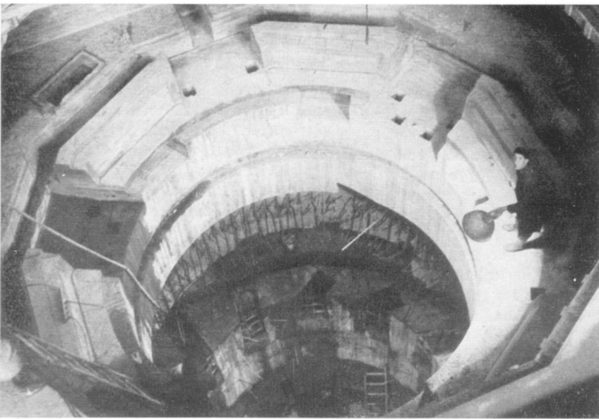
En titt ned i fundamentgraven. Fra ballgolvet til bunnen er det 16,30 meter. Generator og turbin blir forbundet med en vertikal aksling, og det eneste som blir synlig over golvet, er generatorens magnetiseringsmaskin.
