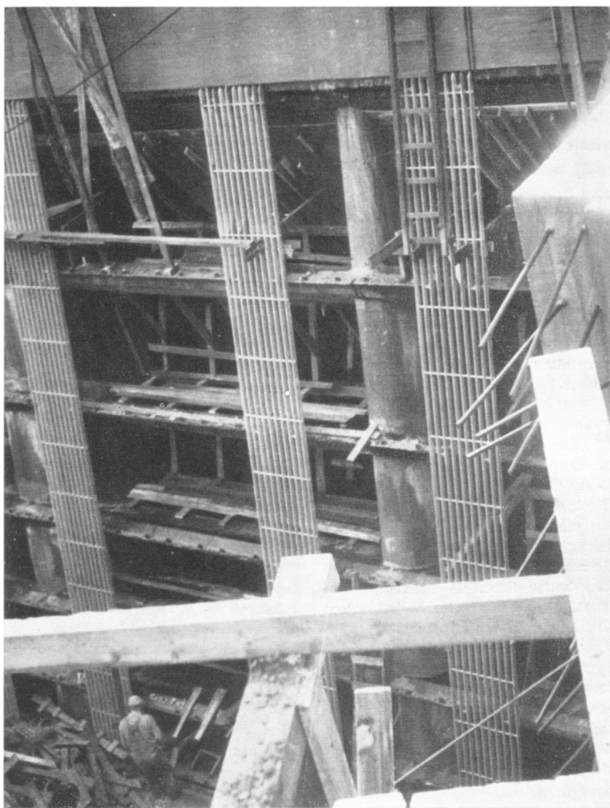
Montasje av varegrindene pågår. Mannen i bunnen gir et inntrykk av dimensjonene.
