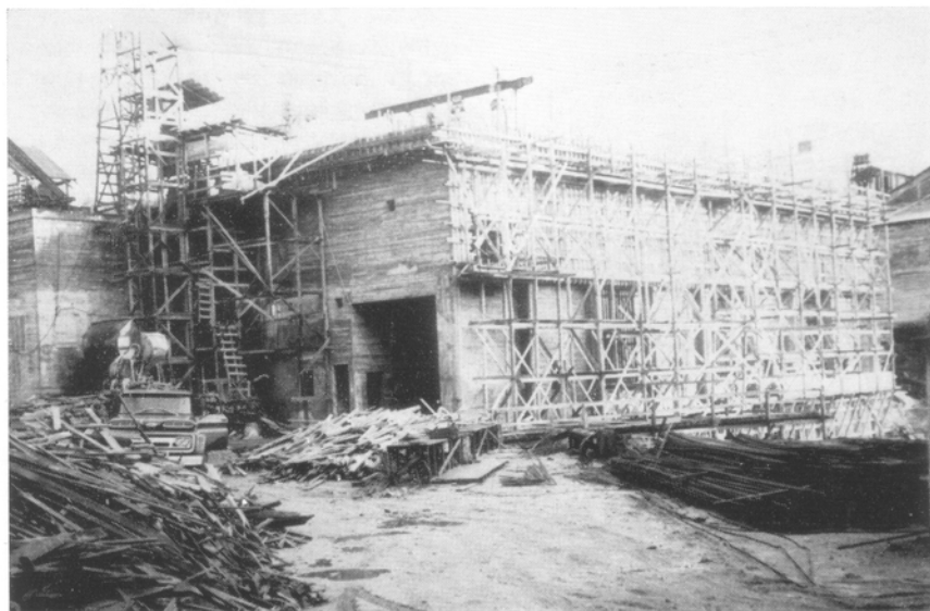
Kraftstasjonen har fått tak på. Jernbanesporet er forlenget helt inn i ballen, slik at maskingodset kan tas direkte fra stasjonsballens egen montasjekran som løfter 60 tonn.
