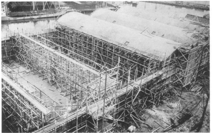
De tre første hvelvene sett fra toppen av Agder Kjøpelags silo. Forskallingen er akkurat ferdig, og plassen under hvelvene ryddes for å gi plass til rørstillasene.
